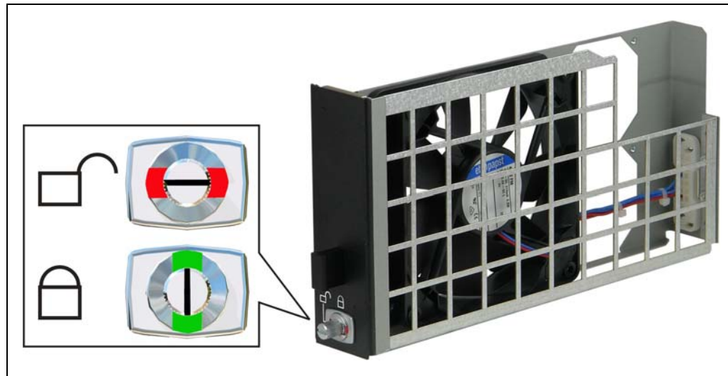
Figure 4: Lüftereinschub
