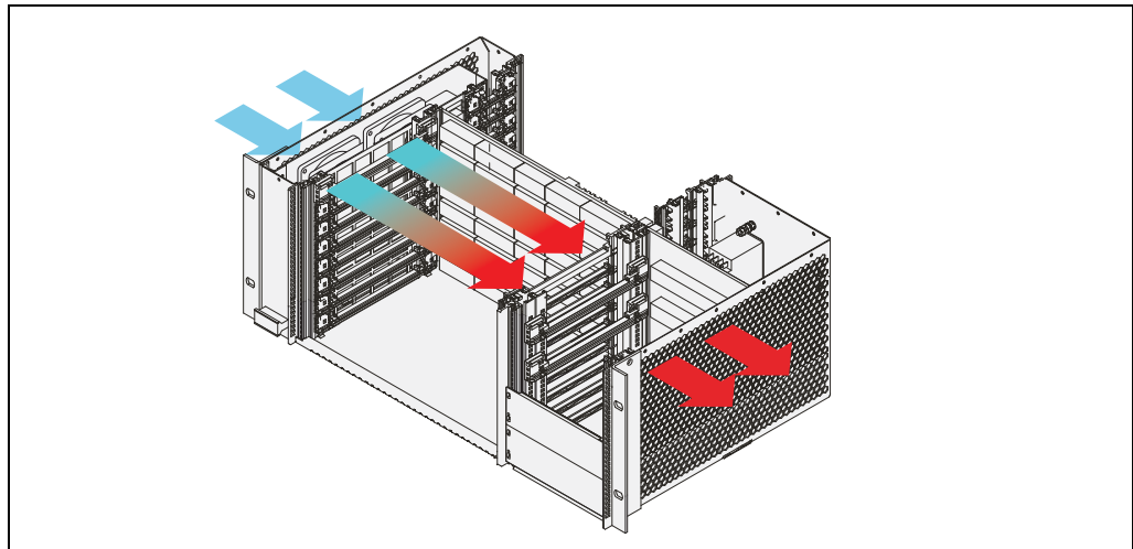
Figure 5: Entwärmung
